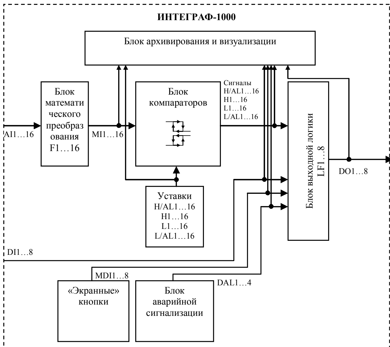
Рисунок 2 – Функциональная структура ИВК ИНТЕГРАФ
