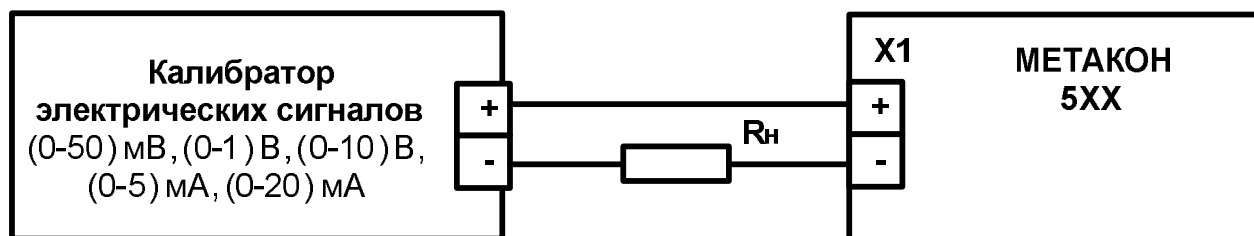
Рисунок А.6.4.1 – Схема подключения приборов мод. МЕТАКОН 5XX для проведения поверки по сигналам напряжения и тока
