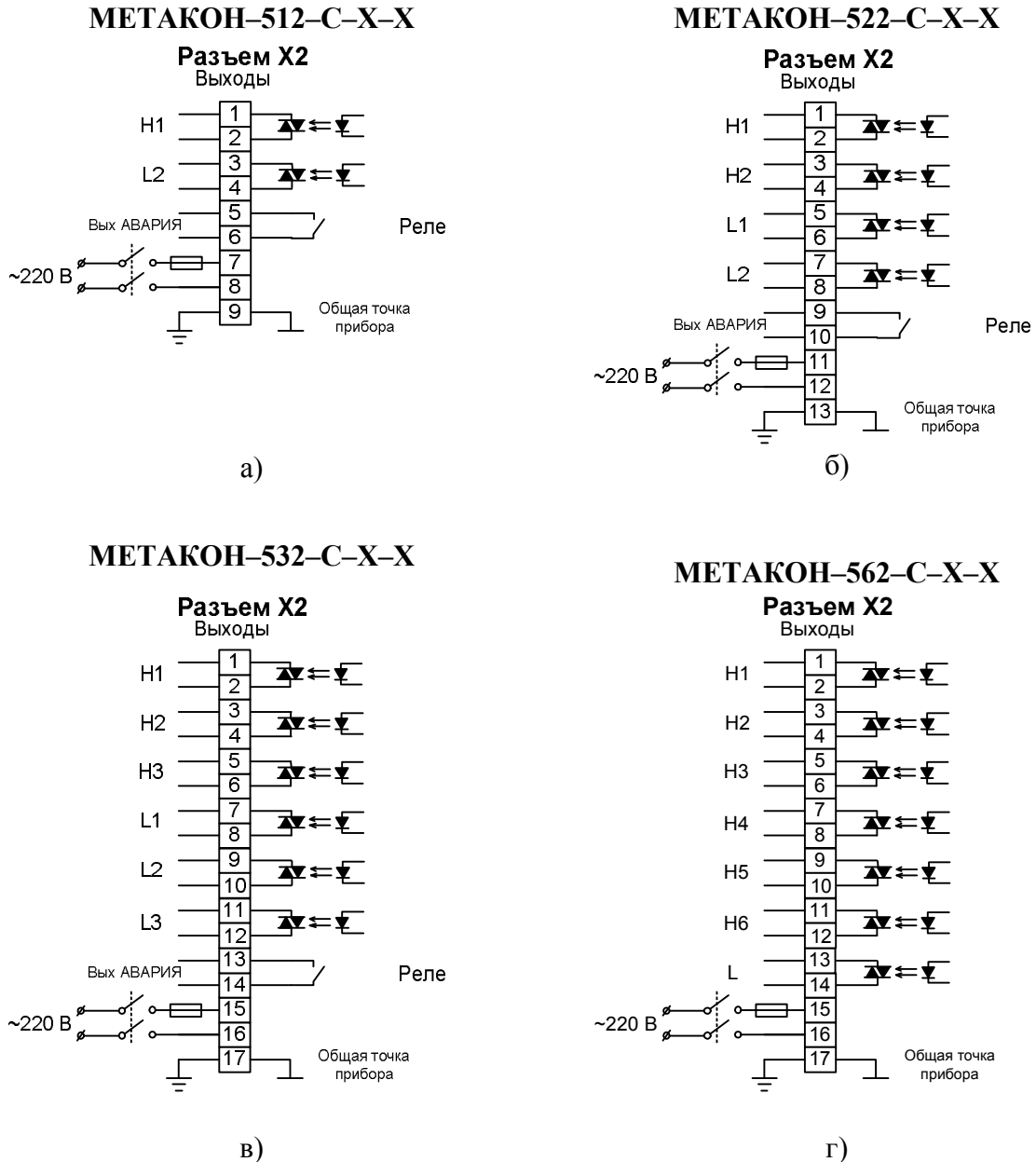
Рисунок 10 – Схемы подключения к клеммным соединителям прибора модификаций МЕТАКОН-5Х2-С-Х
