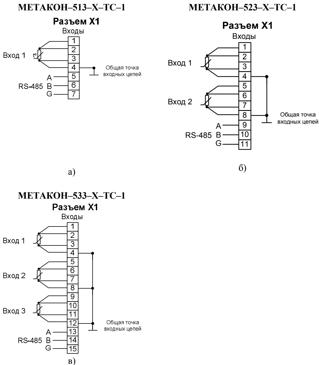
Рисунок 9 – Схемы подключения термопреобразователей сопротивления к клеммным соединителям для мод. МЕТАКОН-5X3-X-ТС-1
