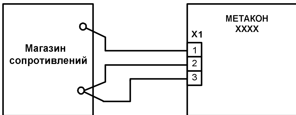
Рисунок А.6.4.1.3 - Схема подключения прибора МЕТАКОН-1105 для проведения поверки по сигналам сопротивления
