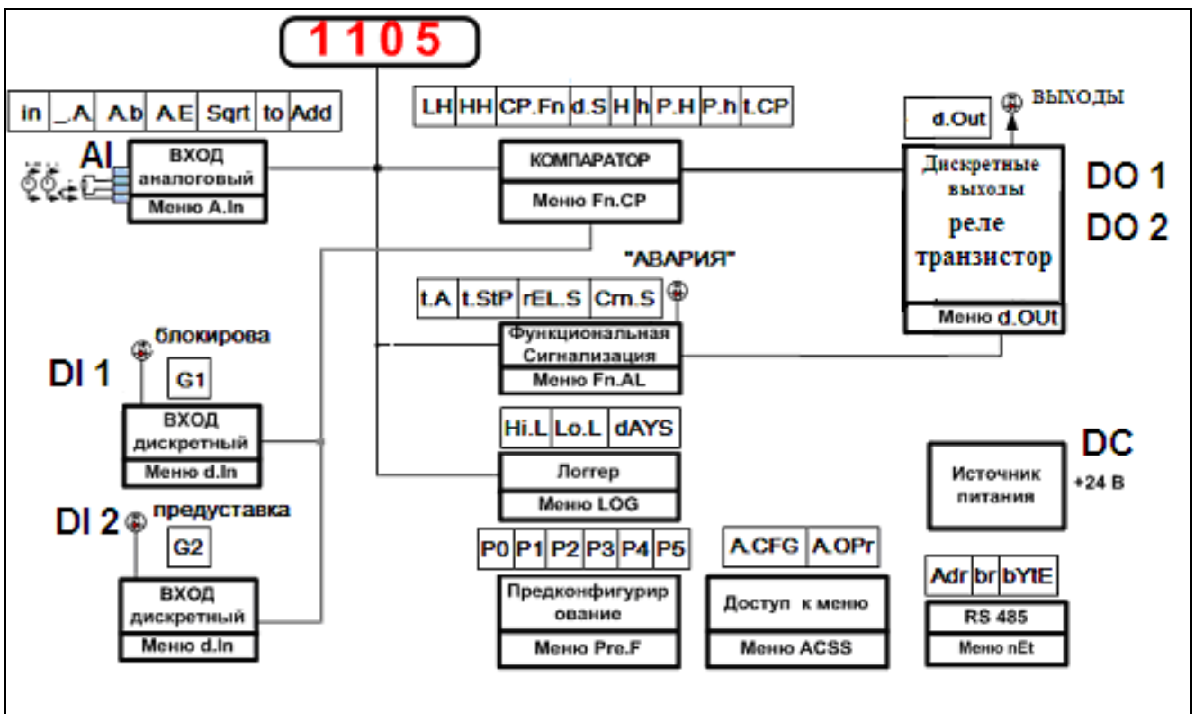
Рисунок 2 – Функциональная схема прибора МЕТАКОН-1105
