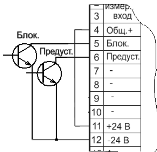
Рисунок 11 – Электрическая схема подключения транзисторов типа N-P-N для управления дискретными входами
