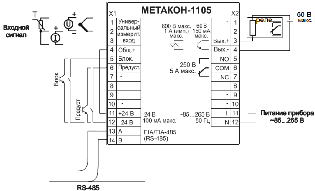
Рисунок 9 – Электрическая схема подключения прибора МЕТАКОН-1105
