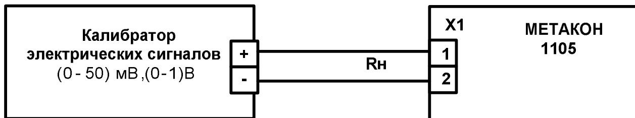
Рисунок А.6.4.1.1- Схема подключения прибора МЕТАКОН 1105 для проведения поверки по сигналам напряжения
