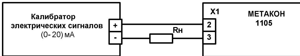
Рисунок А.6.4.1.2 - Схема подключения прибора МЕТАКОН 1105 для проведения поверки по сигналам тока
