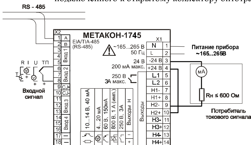
Рисунок 10 – Электрическая схема подключения к прибору МЕТАКОН-1745-2Т/2Р-Y-1 при использовании встроенного источника 24 В для питания внешнего промежуточного реле, подключенного к открытому коллектору оптотранзистора
