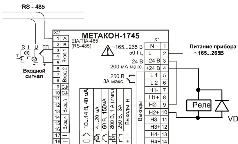
Рисунок 10 – Электрическая схема подключения к прибору МЕТАКОН-1745-2Т/2Р-Y-1 при использовании встроенного источника 24 В для питания внешнего промежуточного реле, подключенного к открытому коллектору оптотранзистора
